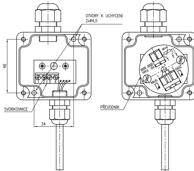
pohled do hlavice snímače do interiéru
