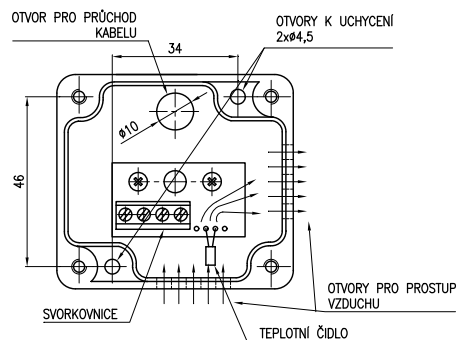
pohled do hlavice snímače do interiéru
