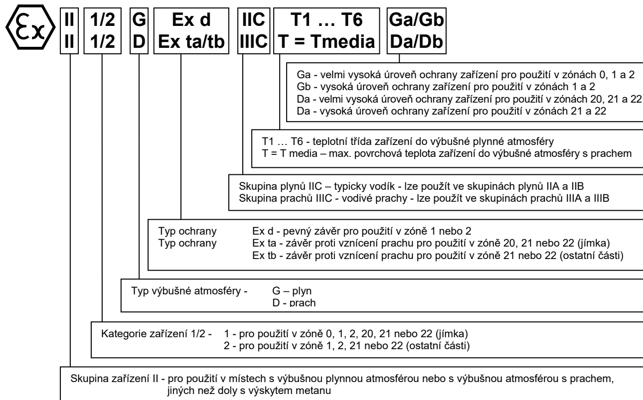
OBRÁZEK 6 - OZNAČENÍ NEVÝBUŠNOSTI
