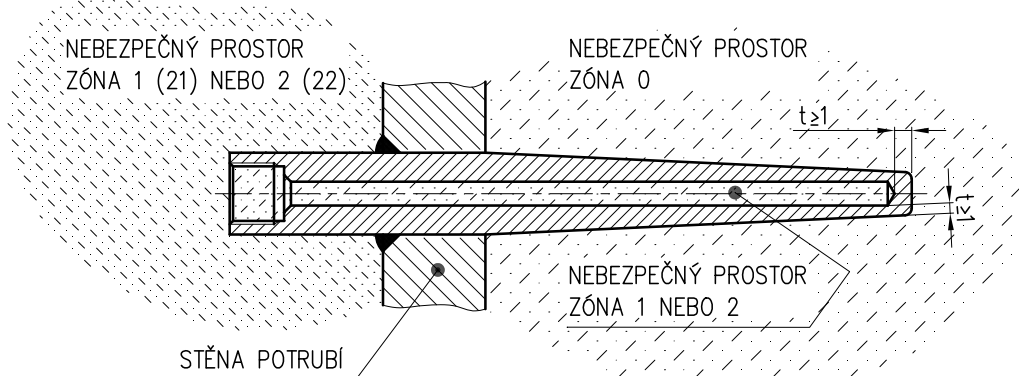
OBRÁZEK 2 – JÍMKA PRO SNÍMAČ TEPLoty Ex d PRO ZÓNU 0 (dle ČSN EN 60079-26 ed. 3)
