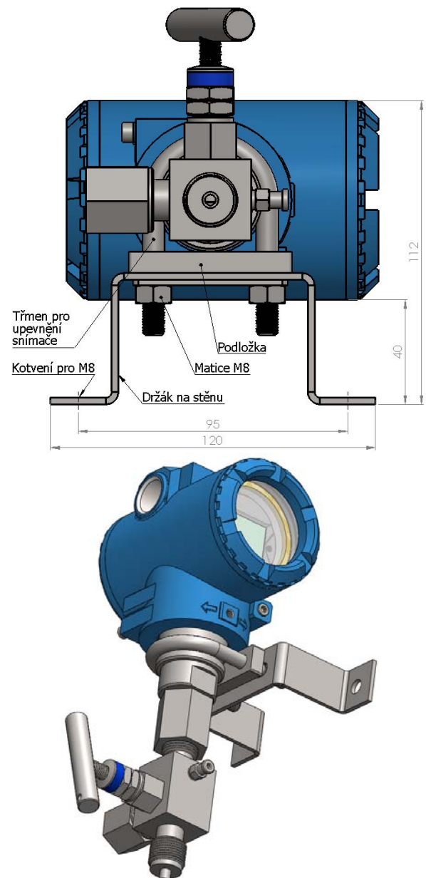
OBRÁZEK 3 - ZPŮSOB MONTÁŽE SNÍMAČE NA STĚNU
