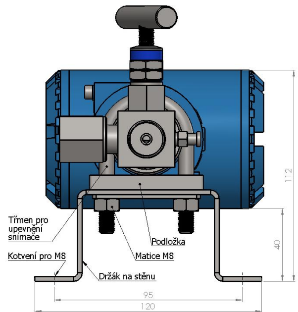
OBRÁZEK 3 - ZPŮSOB MONTÁŽE SNÍMAČE NA STĚNU
