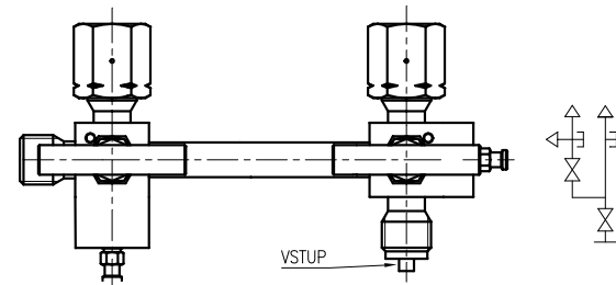
Obrázek 3 – Ventilová jednotka s elastomerovým o-kroužkem
