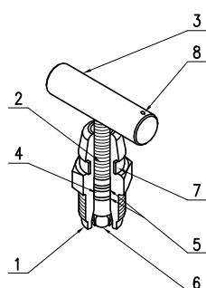
Obrázek 3 – Ventilová jednotka s elastomerovým o-kroužkem
