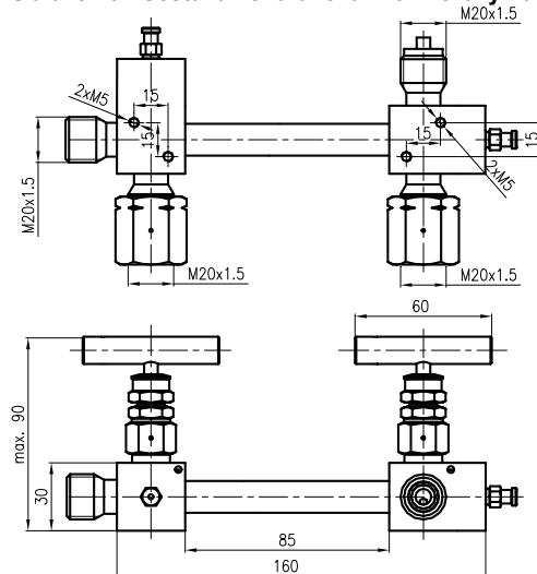
Obrázek 5 – Sestava ventilů levá - rozměrový náčrt
