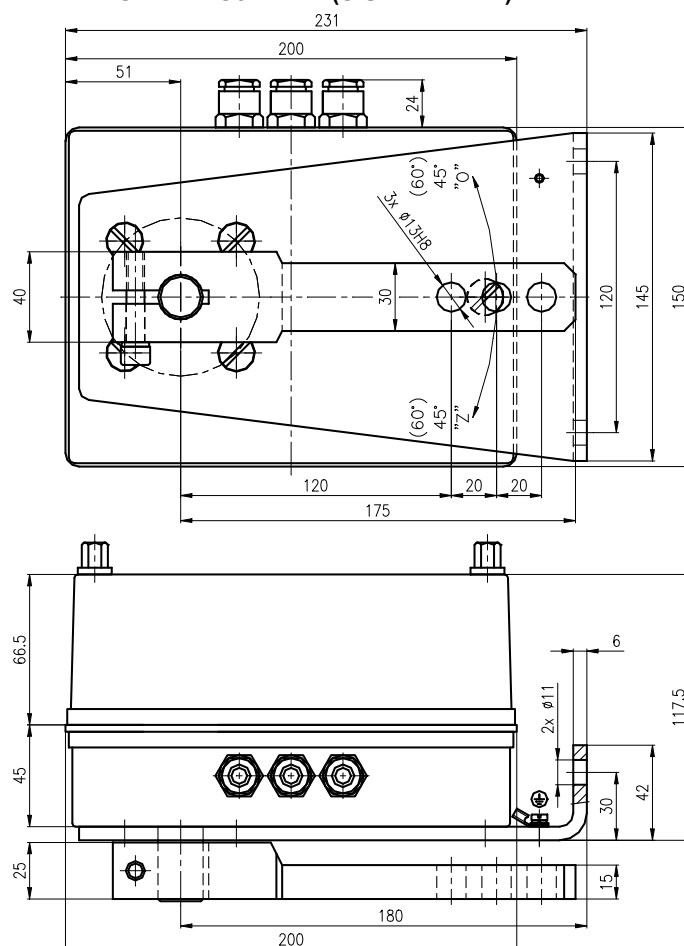
OBRÁZEK 2 - ROZMĚROVÝ NÁKRES – PŘIPOJENÍ P31 AŽ P38 (BEZPŘÍRUBOVÉ UZAVÍRACÍ Klapky)
