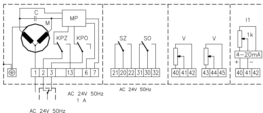
SCHEMA ZAPOJENÍ 24V 50Hz
