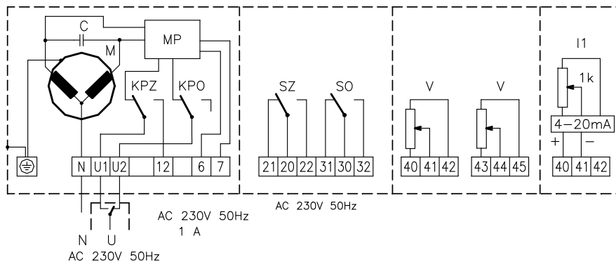
SCHEMA ZAPOJENÍ 230V 50Hz
