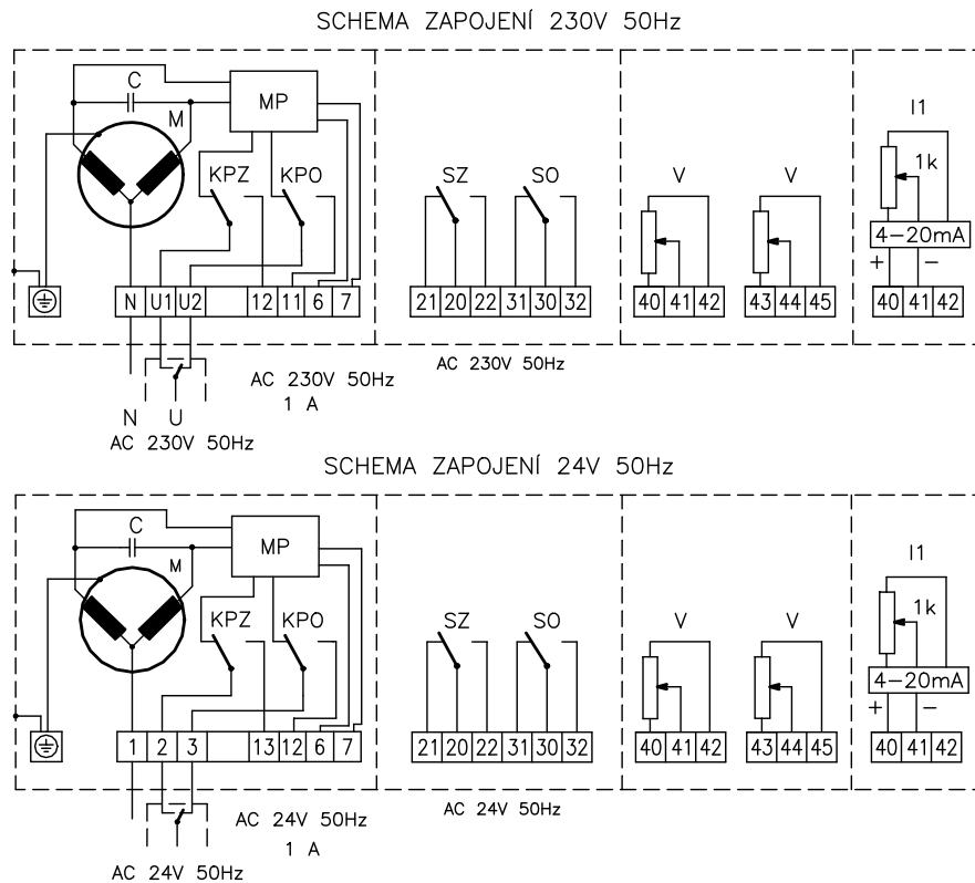
OBRÁZEK 4 - SCHÉMA ZAPOJENÍ A NÁKRES SVORKOVNICE - TŘÍBODOVÉ ŘÍZENÍ S MOMENTOVOU POJISTKOU
