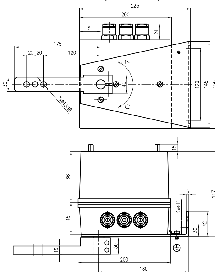
OBRÁZEK 2 - ROZMĚROVÝ NÁKRES – PŘIPOJENÍ P31 AŽ P38 (BEZPŘÍRUBOVÉ UZAVÍRACÍ KLAPKY)
