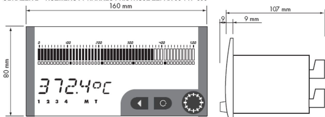
OBRÁZEK 2 – ROZMĚROVÝ NÁKRES PŘÍSTROJE ZEPAX 06 TYP 506
