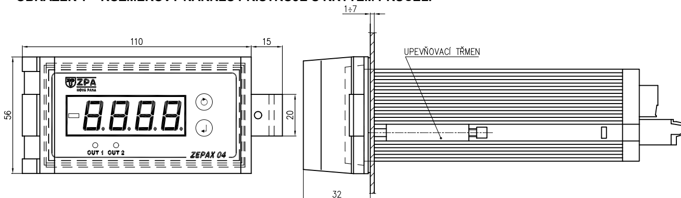
OBRÁZEK 1 – ROZMĚROVÝ NÁČRT PŘÍSTROJE S KRYTEM PRŮČELÍ
