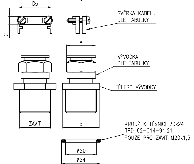
Obrázek 1- Rozměrový náčrtek
