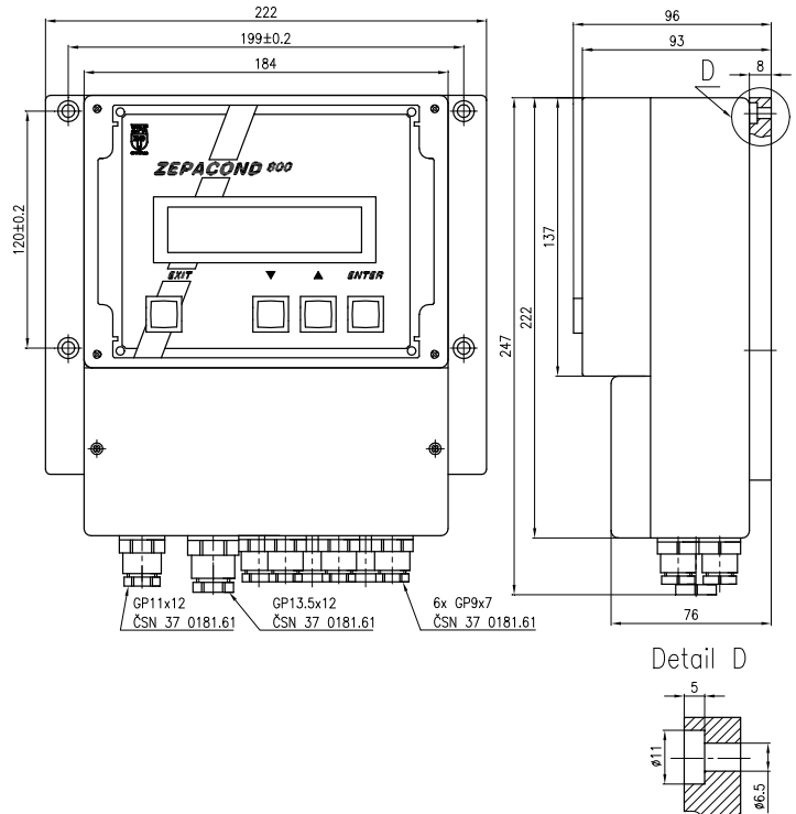
OBRÁZEK 1 - ROZMĚROVÝ NÁKRES
