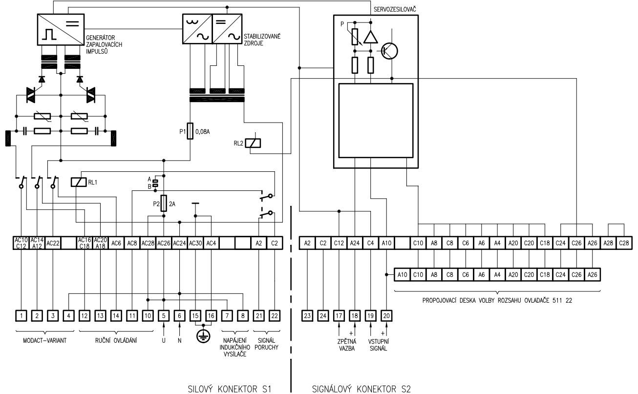
OBRÁZEK 6 - BLOKOVÉ SCHÉMA OVLADAČŮ 511 21 A 511 22 S PROUDOVOU ZPĚTNOU VÁZBOU
