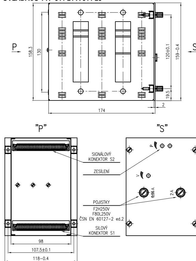
OBRÁZEK 2 - ROZMĚROVÝ NÁKRES OVLADAČŮ VE SKŘÍNI TYP 511 22 A 511 26
