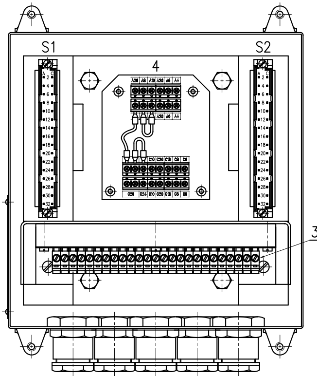
OBRÁZEK 3 - NÁKRES UMÍSTĚNÍ KONEKTORŮ, SVORKOVNICE A PROPOJOVACÍ LIŠTY VE SKŘÍNI OVLADAČŮ TYP 511 22 A 511 26
