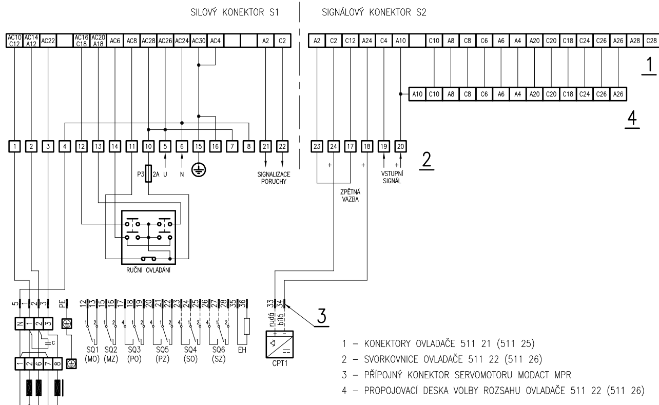
OBRÁZEK 4 - SCHÉMA PŘIPOJENÍ OVLADAČŮ SE SERVO MOTOREM V PROVEDENÍ "KONEKTOR"
