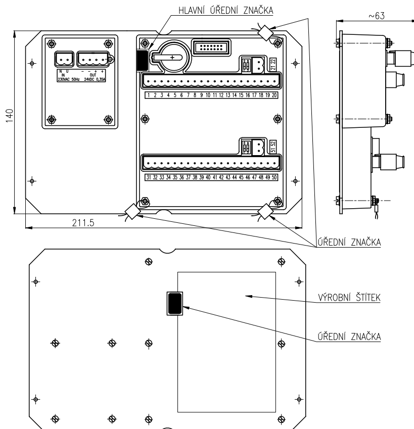
OBRÁZEK 3 - UMÍSTĚNÍ ÚŘEDNÍCH ZNAČEK A VÝROBNÍHO ŠTÍTKU NA KAZETĚ
