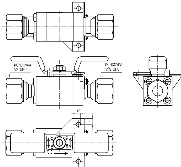
OBRÁZEK 6 KOHOUT KULOVÝ - PŘÍKLAD SPECIÁLNÍ ÚPRAVY - ZÁVITY PRO PŘIPEVNĚNÍ NA STĚNU NEBO NA DRŽÁK (971 .. D1), ROZMĚROVÝ NÁKRES
