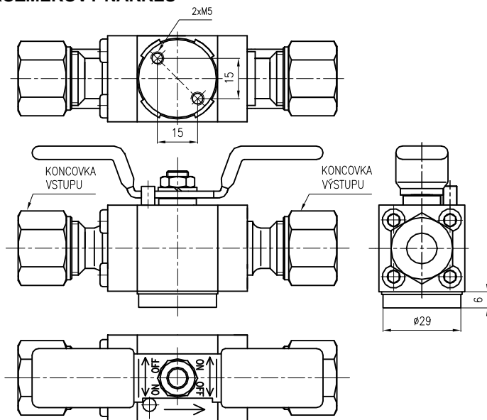
OBRÁZEK 6 KOHOUT KULOVÝ - PŘÍKLAD SPECIÁLNÍ ÚPRAVY - ZÁVITY PRO PŘIPEVNĚNÍ NA STĚNU NEBO NA DRŽÁK (971 .. D1), ROZMĚROVÝ NÁKRES
