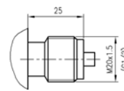
nákres šroubení
