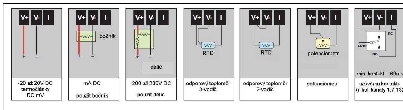
OBRÁZEK 7: ZAPOJENÍ VSTUPNÍCH SIGNALŮ
