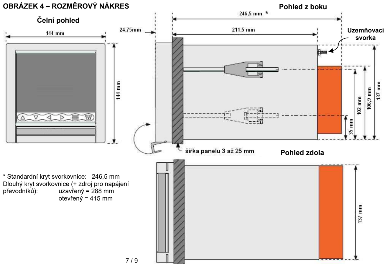
OBRÁZEK 4 – ROZMĚROVÝ NÁKRES
