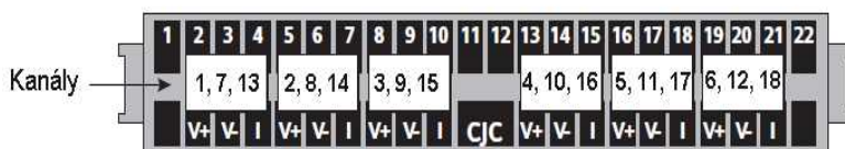
OBRÁZEK 6 - ZAPOJENÍ VSTUPNÍCH KANÁLŮ
