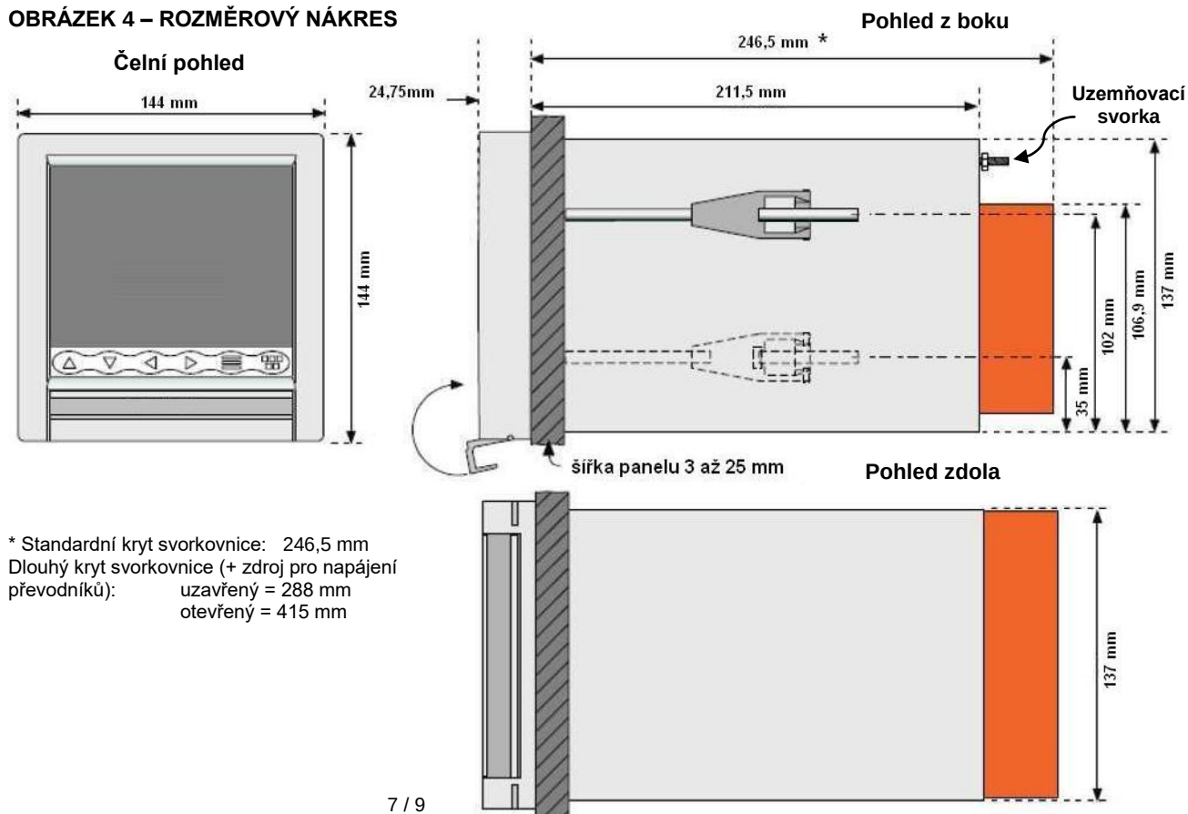
OBRÁZEK 4 – ROZMĚROVÝ NÁKRES
