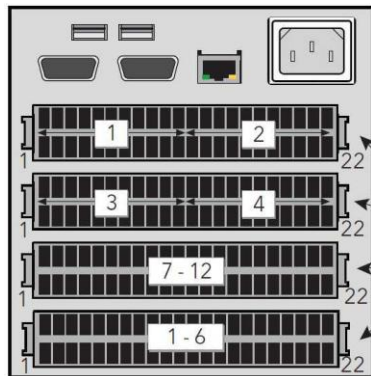
OBRÁZEK 5 - USPOŘÁDÁNÍ SVORKOVNICE
