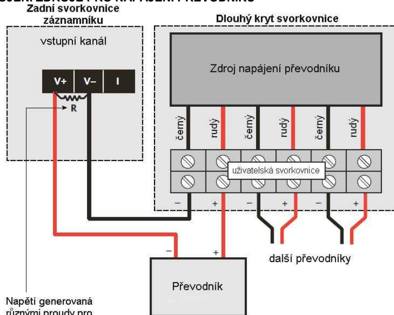
OBRÁZEK 11 - ZAPOJENÍ ZDROJE PRO NAPÁJENÍ PŘEVODNÍKU
