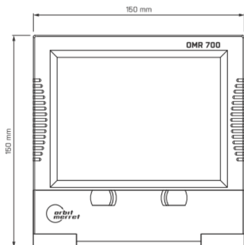
OBRAZEK 3 – ROZMĚROVÝ NÁKRES
