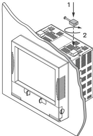
OBRAZEK 2: VÝŘEZ V PANELU
